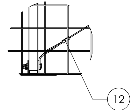
Detail V 1 : 10
